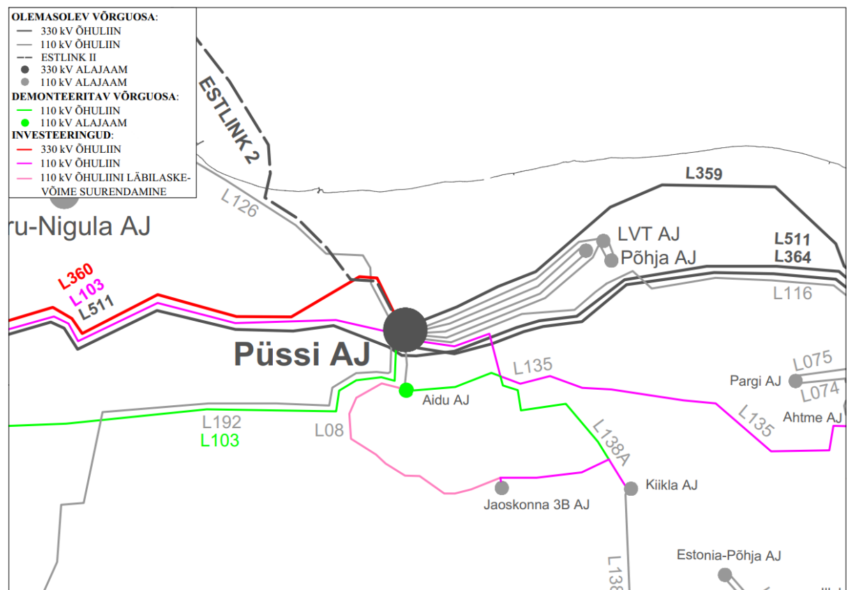
Joonis 11. Muutused 110 kV elektrivõrgus Lüganduse vallas 2030.a perspektiivis.
