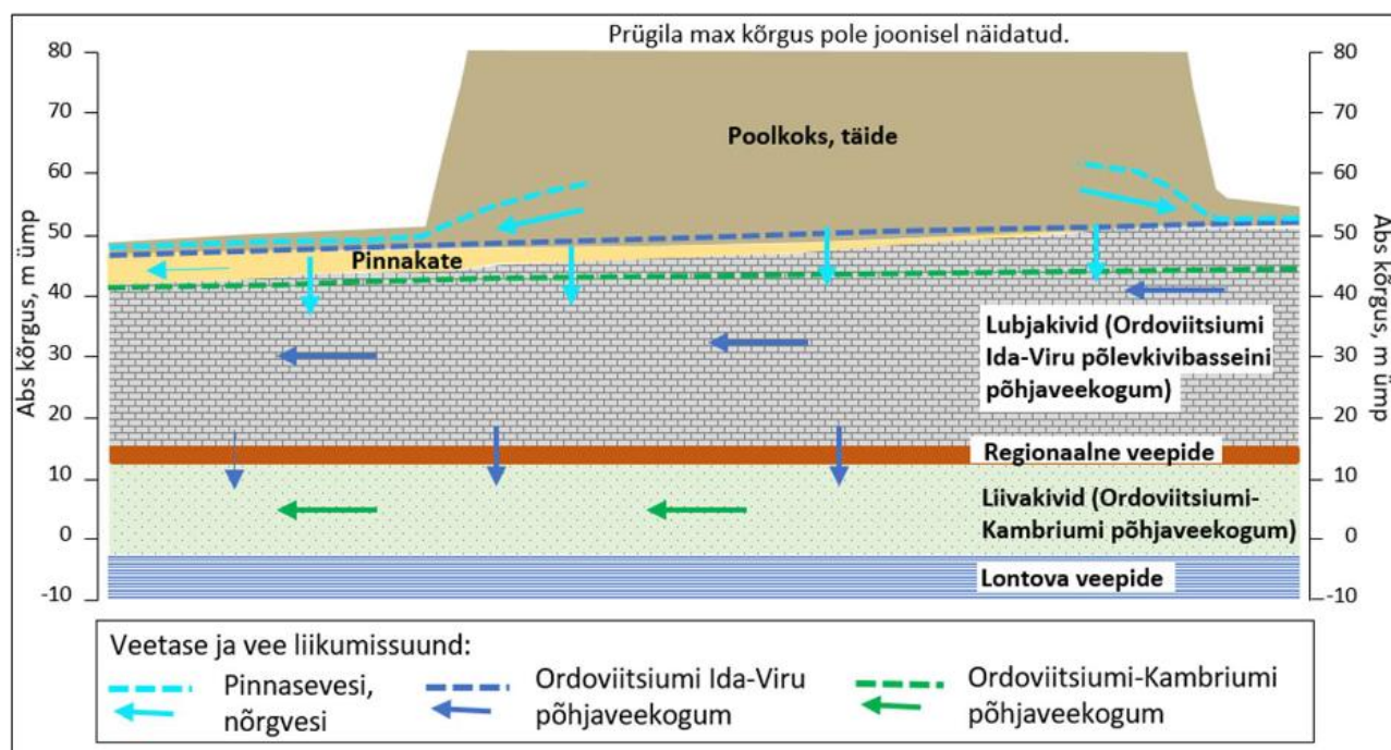
Joonis 17. Olemasoleva tööstusjäätmete ala ja lähiümbruse (iseloomustab ka piirnevat planeeringuala) skemaatiline ida-lääne-suunaline geoloogiline läbilõige (IPT Projektijuhtimine OÜ, 2023).
