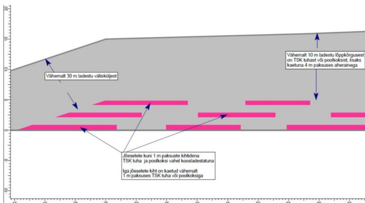
Joonis 37. Jõesetete „kärgedesse“ ladestamise põhimõtteline skeem (OÜ IPT Projektijuhtimine, 2019).
