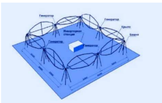
Joonis 3 Taastuenergiaparki kavandatud mikrotuulikud WTW-01.001
