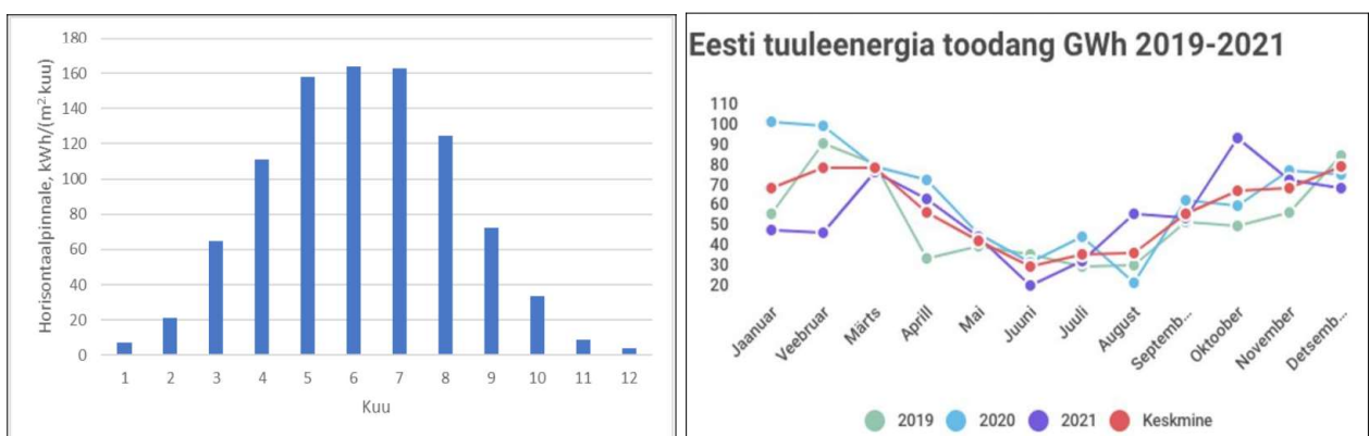
Joonis 10 Päikeseenergia (Hevac 2020) ja tuuleenergia (Eesti Taastuenergia Assotsiatsioon 2022) efektiivne tootlikus Eestis, kuude lõikes
