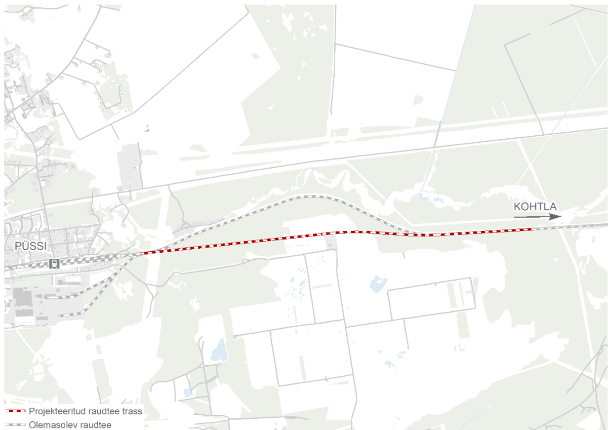
Joonis 10. Projekteeritud raudtee trass.
